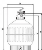
Cantabric Top szűrőtartály
