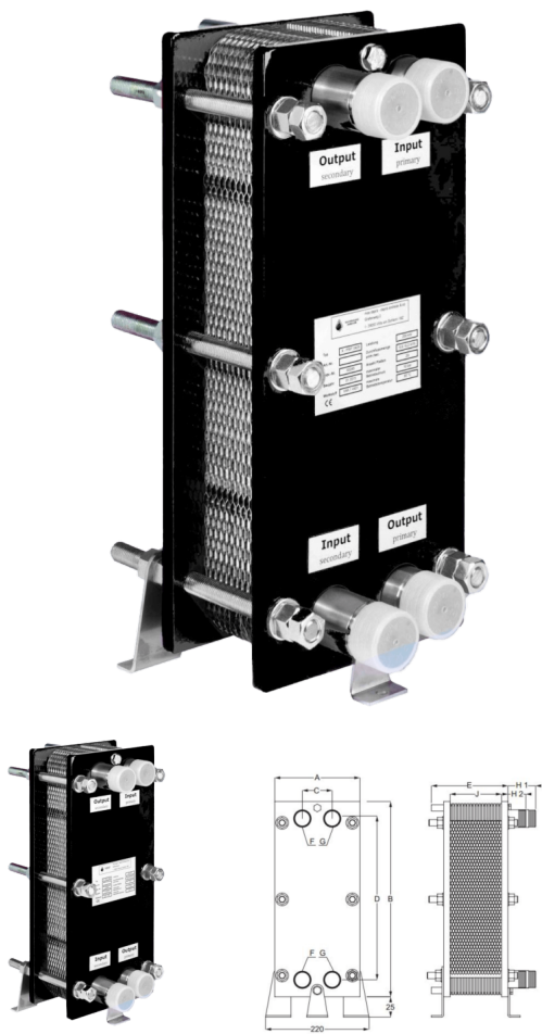
Lemezes hűtőcserél? Power X-PWT 419-VA - 135 kW - 70°C
