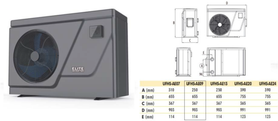
Elite Inverter hőszivattyú
