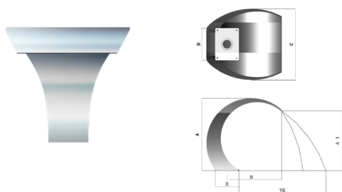
Cobra 400 AISI316 LC D50 Nyakzuhany
