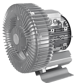
Légfűvő 710T 3,0kW/400V, 318m 3 /h 270mbar
