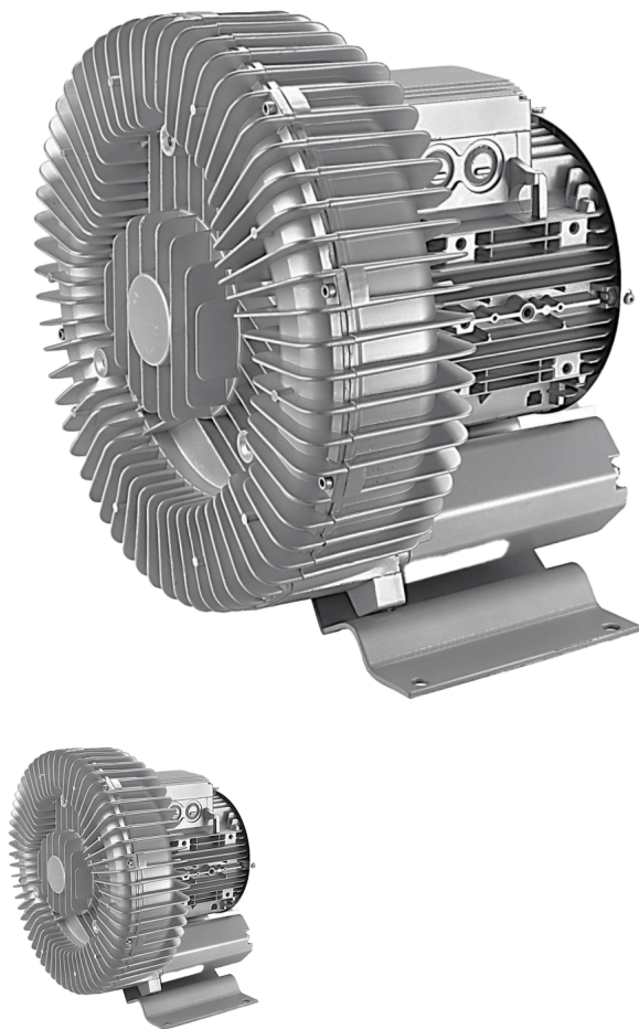
Légfűvő 310T 0,7kW/400V, 100m 3 /h 150mbar
