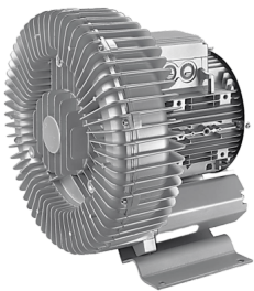
Légfűvő 430T 1,3kW/400V, 180m 3 /h 180mbar
