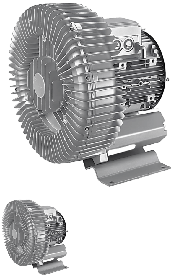
Légfűvő 740T 5,5kW/400V, 530m 3 /h 300mbar
